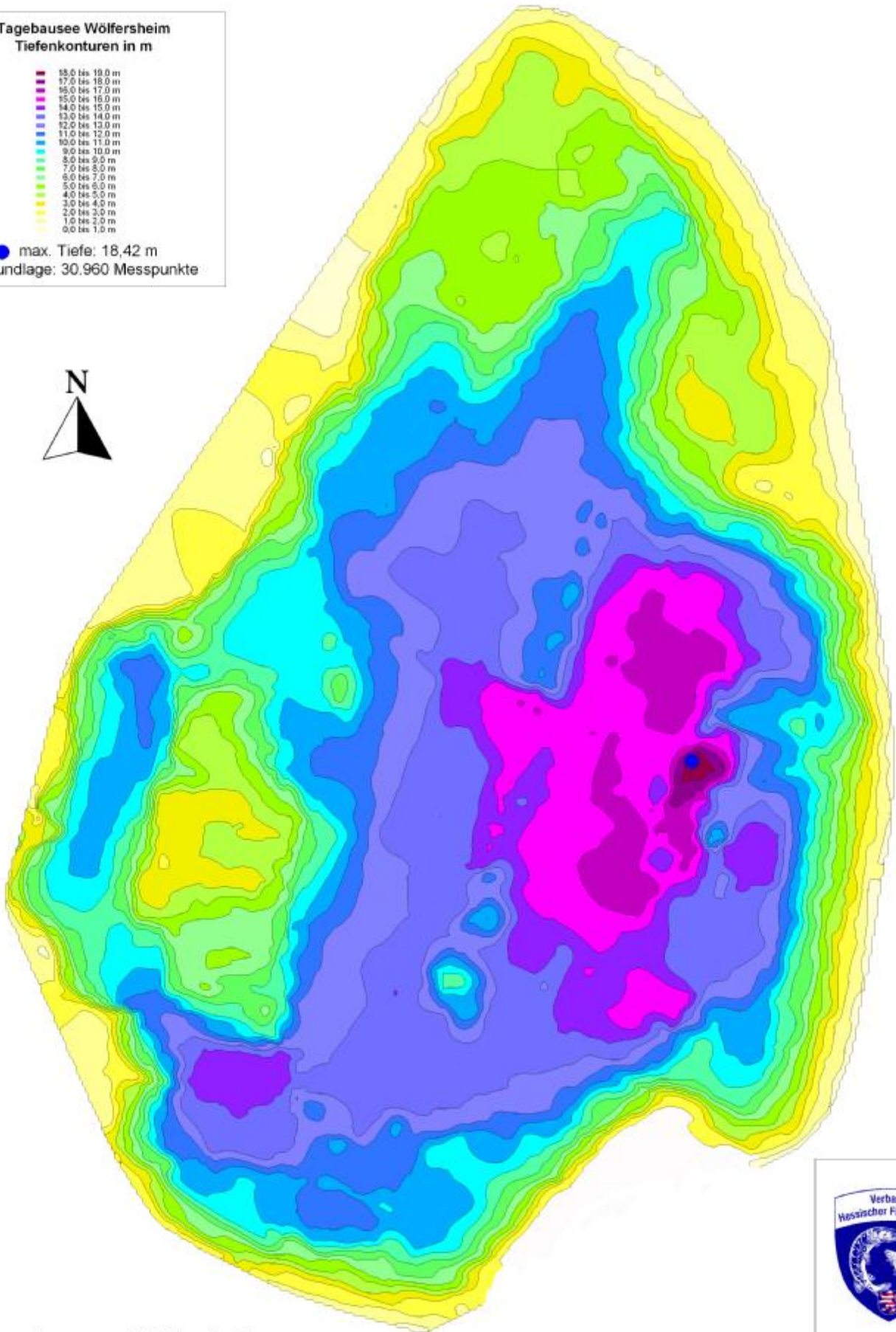
Tagebausee Wölfersheim Echographenfahrt am 13.9.2008: Tiefenkonturen 1 m
